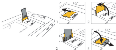
Rysunek12. Wkładanie karty multimedialnej
